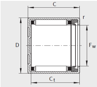
BK...-RS 其 F_w \geq 25\text{ mm}
