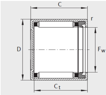
BK...-RS 其 F_w < 25\text{ mm}
